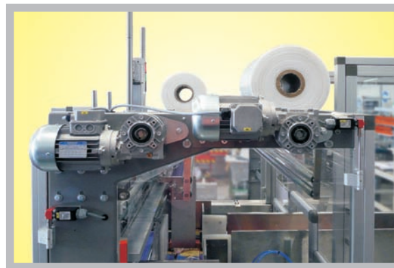
Doppel-Folienlager oben Double film stock on top Magasin de film double au-dessus
