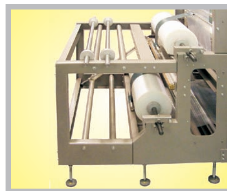
Seitlich angeordnetes Folienlager zur Aufnahme von 4 Folienrollen Laterally installed film support for the retaining of 4 film rolls Support film latéral pour recevoir 4 bobines de film
